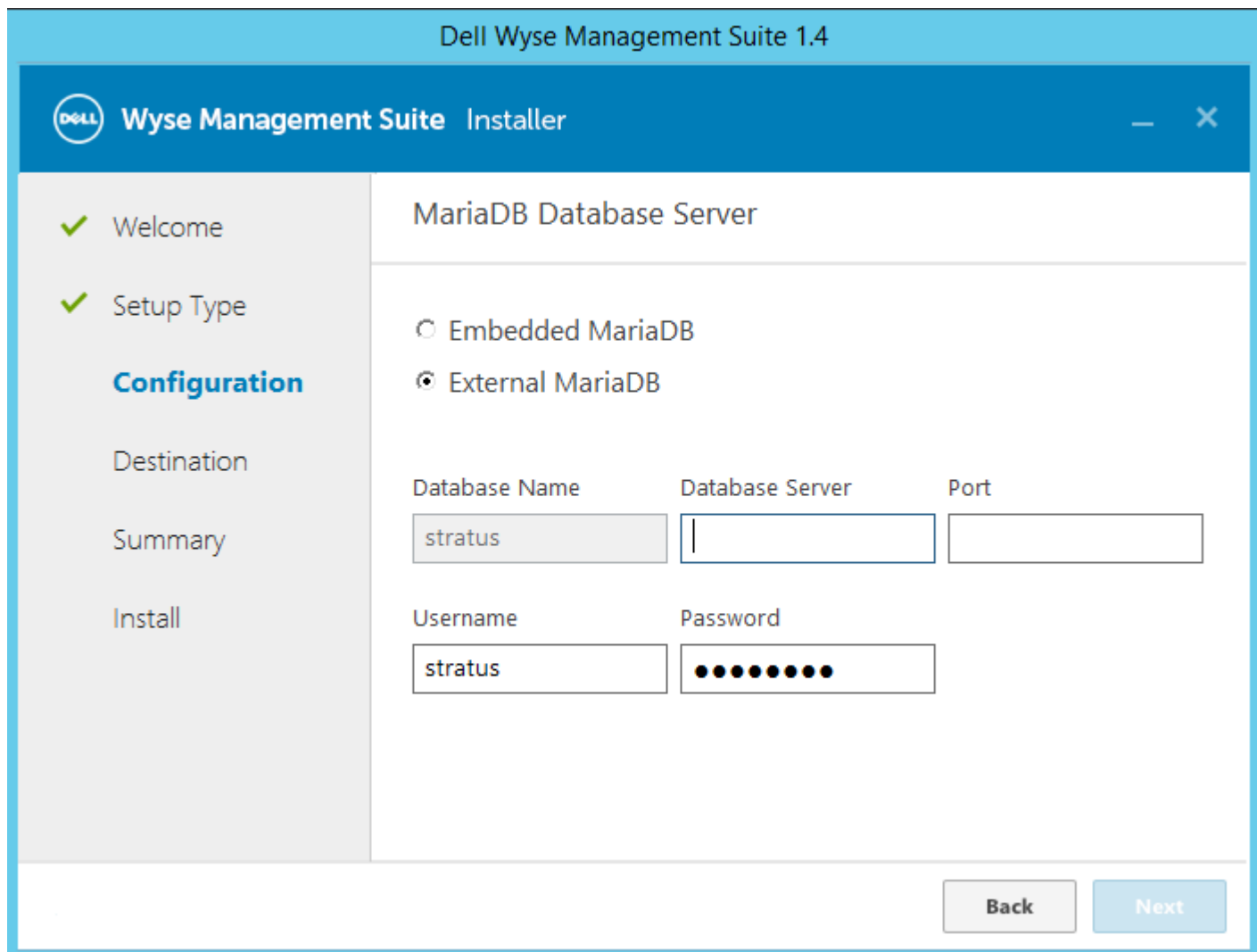
图 22: 外部 MariaDB
